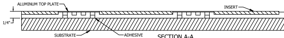
SECTION A-A SCALE 1:1
