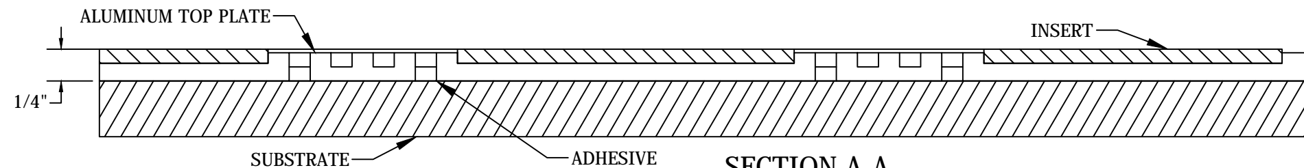
SECTION A-A SCALE 1:1
