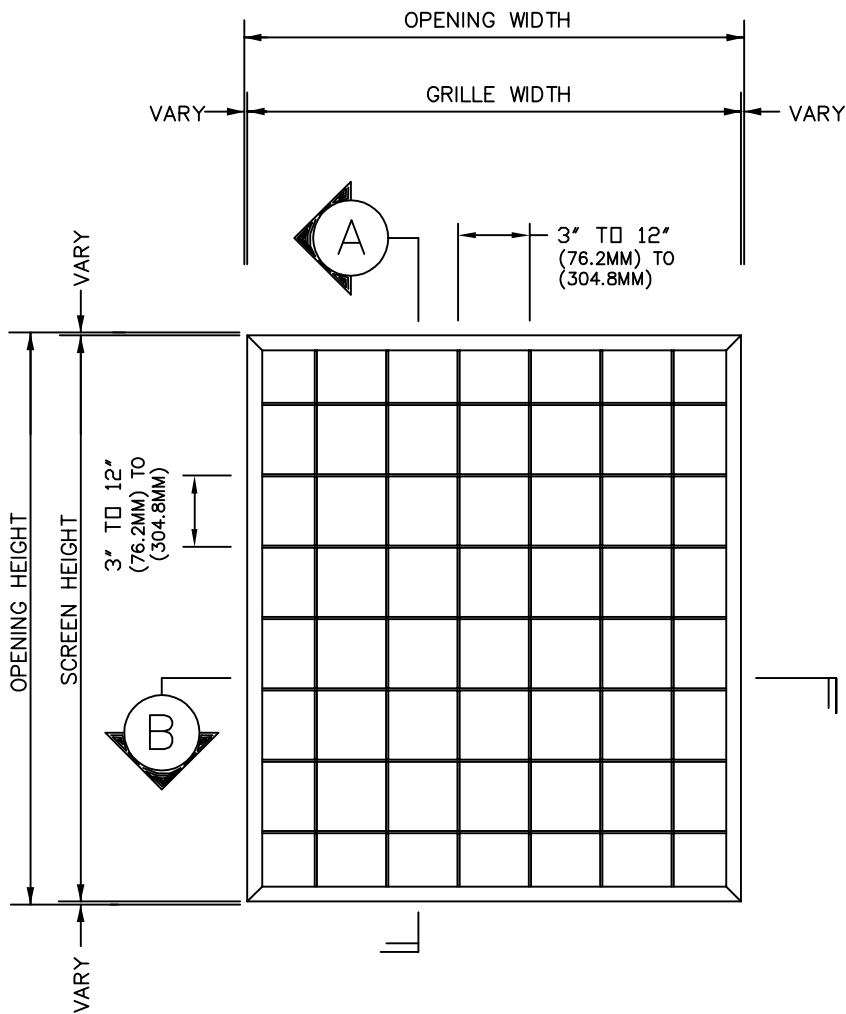
ELEVATION
