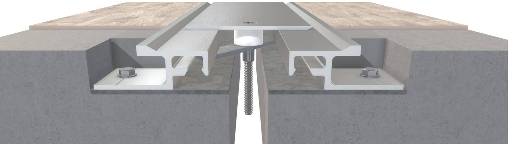
Model SJPF
