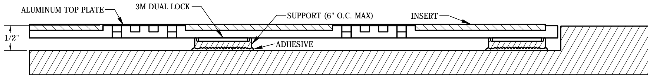
SECTION A-A SCALE 1:1
