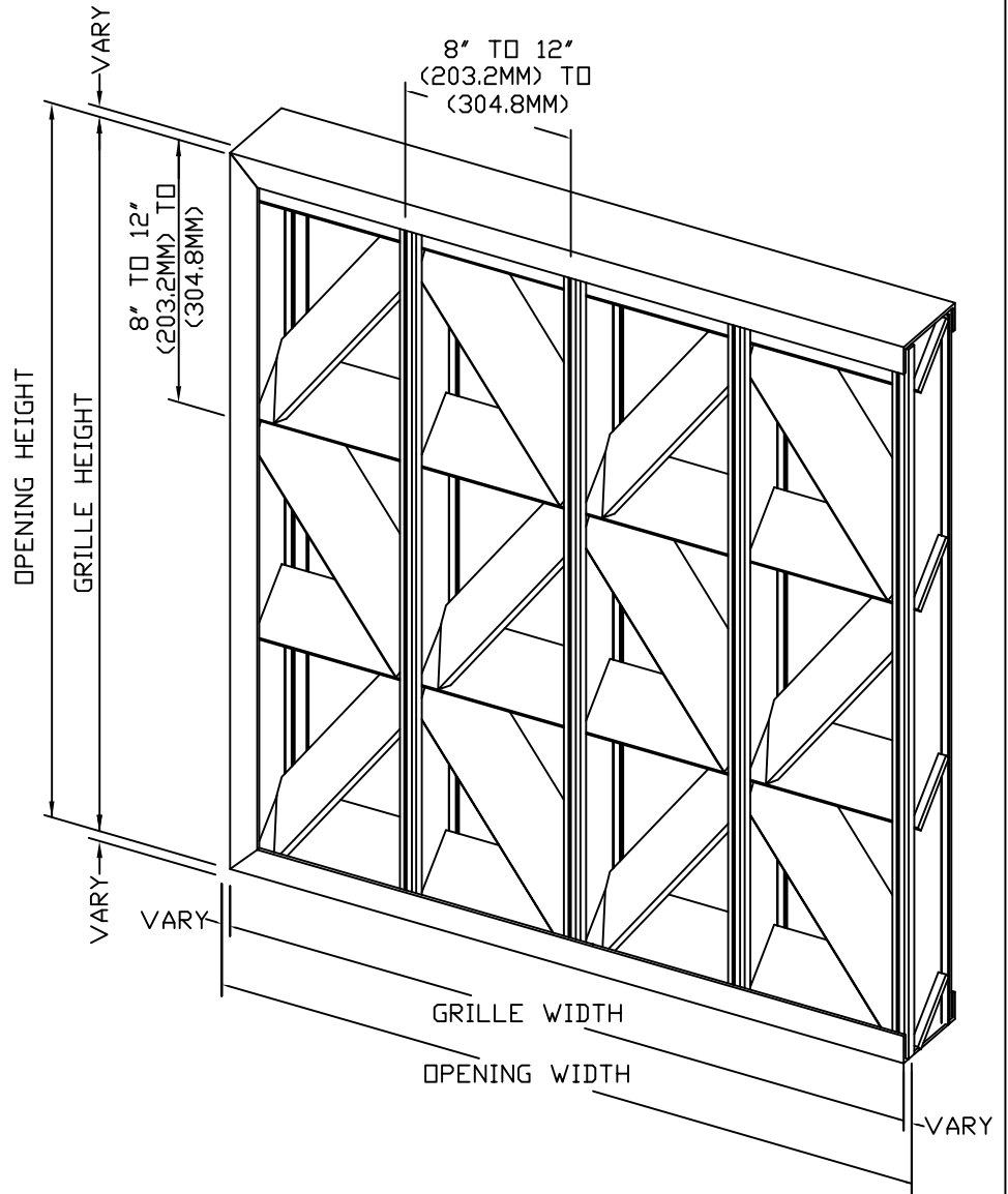
ELEVATION
