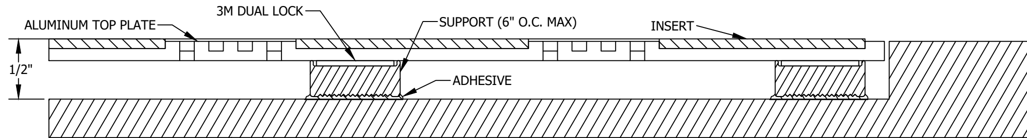
SECTION A-A SCALE 1:1
