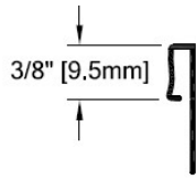
Moldura de zócalo (25N036xxxS, para hoja de .040/.060") (25N040xxxS, para hoja de .075")
