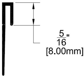
Moldura para parte baja de pared (25A023XXX)
