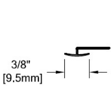
Moldura vertical (25N033xxxS, para hoja de .040/.060") (25N038xxxS, para hoja de .075")
