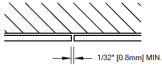
Junta vertical estándar Consulte la tabla de movimiento térmico para conocer el espaciado adecuado.
