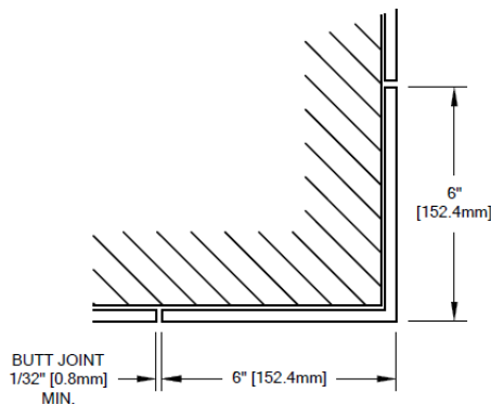
Moldura de esquina exterior conformada
