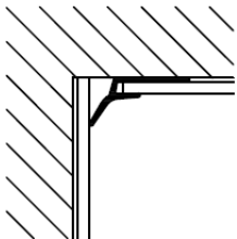
Moldura de esquina interior estándar para exteriores
