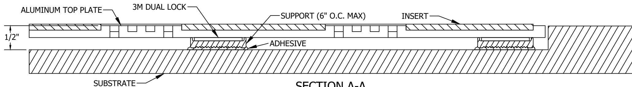
SECTION A-A SCALE 1:1
