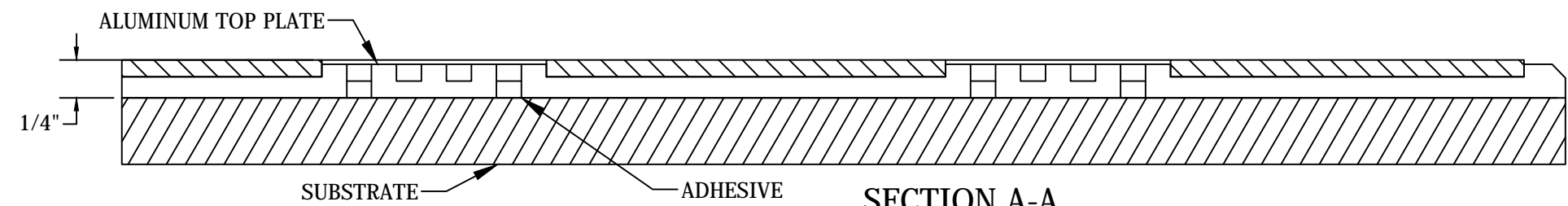
SECTION A-A SCALE 1:1
