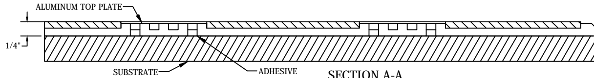
SECTION A-A SCALE 1:1
