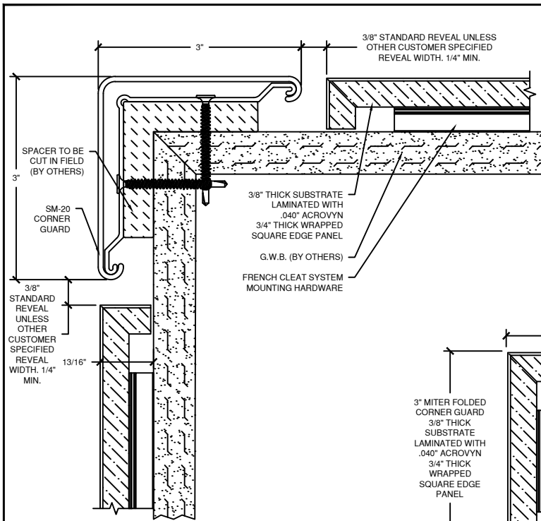
(D) SM-20 OUTSIDE CORNER OPTION
